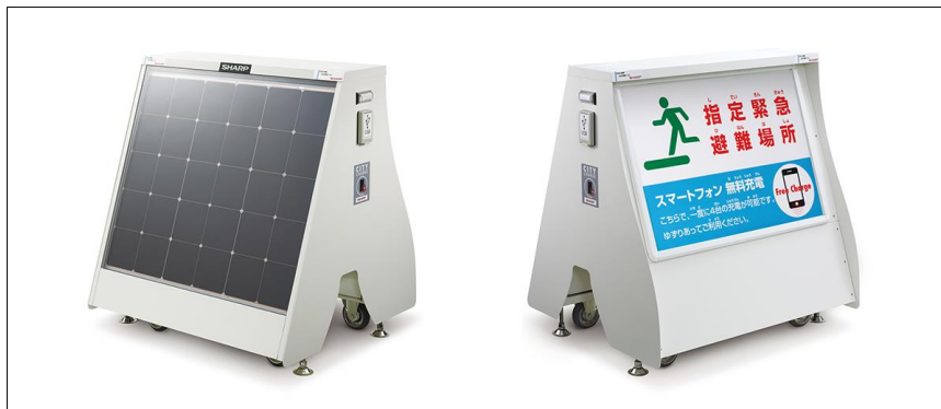
シャープ 移動可能型ソーラー充電スタンド<LN-CB1AA> (左：太陽光パネル側、右：掲示板上側)
