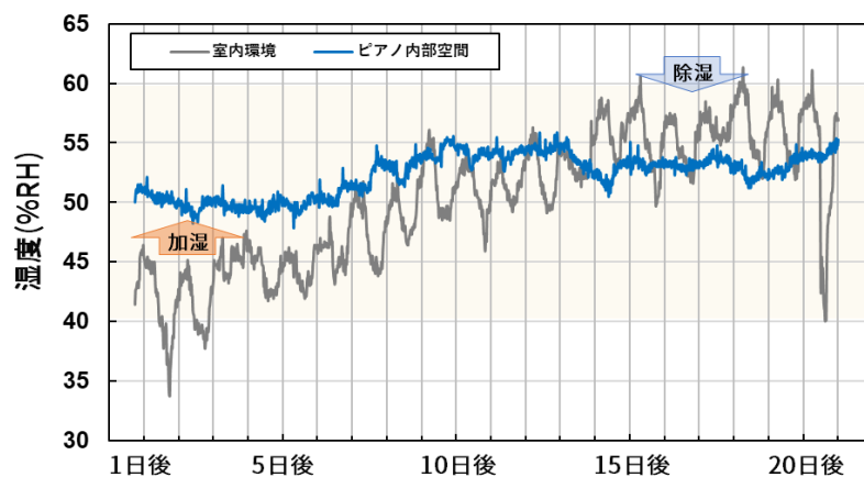
湿度調整剤EMUL 『EML-TKJN01』使用時のアップライトピアノ内部での調湿実験の結果※2 (環境湿度に対するピアノ内部の湿度変化)
