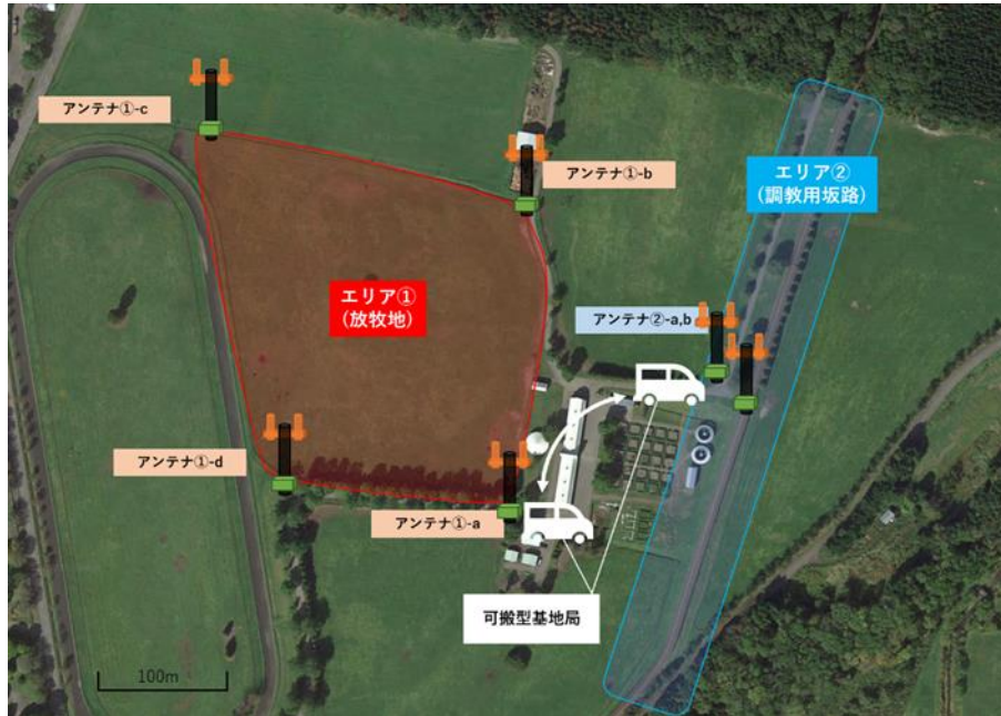
分散アンテナシステムによるローカル5Gエリア構築 (放牧地に加え、調教用坂路にも設置。可搬型基地局の移動で両エリアの通信制御に対応)
